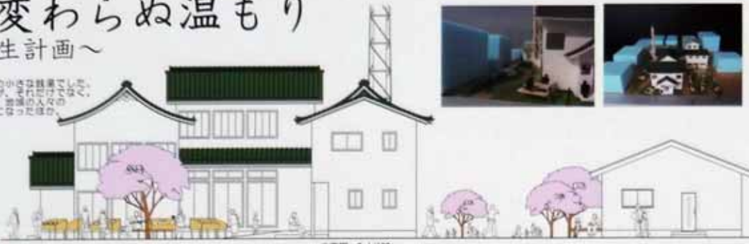
立面図 1/100
