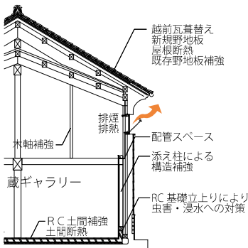
蔵ギャラリー断面詳細図
