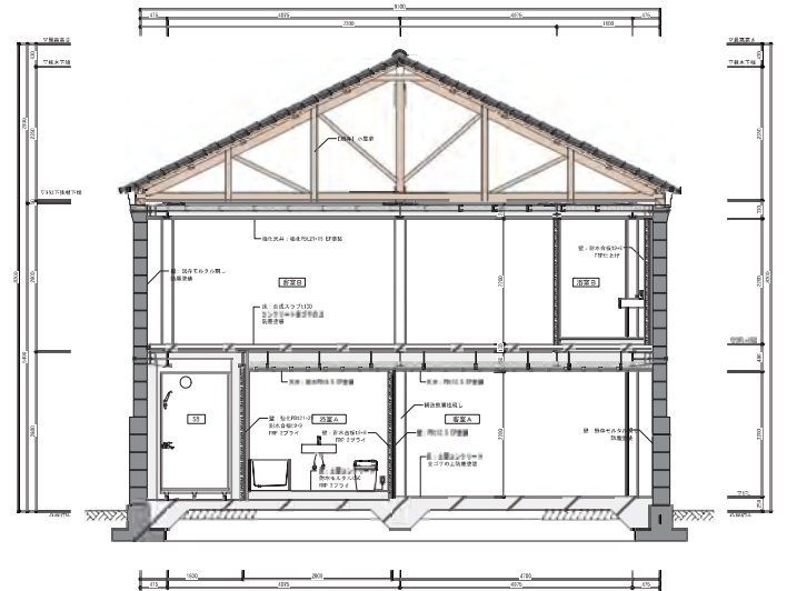
矩計図
