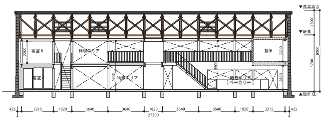
改修断面図
